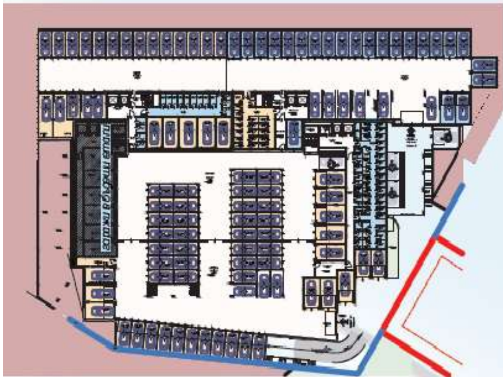
РАЗПРЕДЕЛЕНИЕ ГАРАЖИ ЕТАЖ -2
