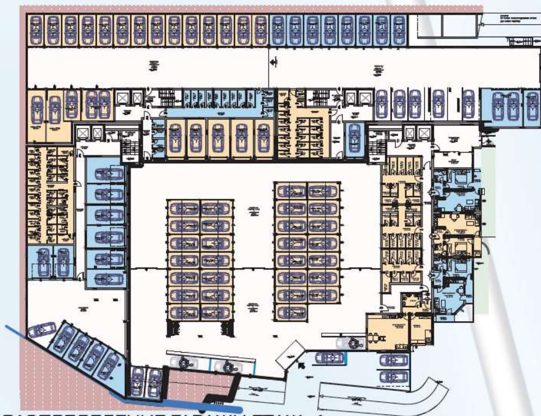
РАЗПРЕДЕЛЕНИЕ ГАРАЖИ ЕТАЖ -1
